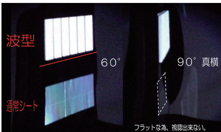
波型形状の反射材は真横からの光にも再帰反射します
